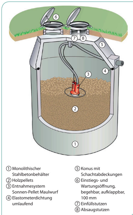
1 Unterirdischer Holzpelletspeicher mit oberer Entnahme
