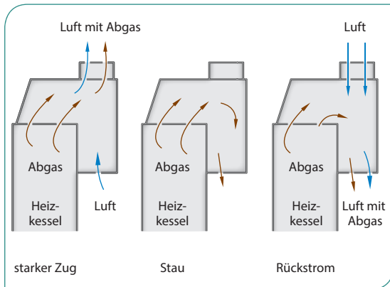
3 Integrierte Strömungssicherung
