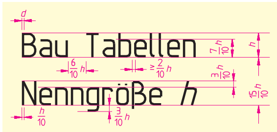
Maße der Schriftform B, vertikal (V) nach DIN EN ISO 3098-1 (Abstand zwischen Schriftzeichen von zwei Linienbreiten zur Sicherstellung der Lesbarkeit; Verringerung des Abstandes auf eine Linienbreite, wenn Schriftzeichen wie z.B. TV, LA zusammentreffen, um ein gutes Schriftbild zu erzielen.)
