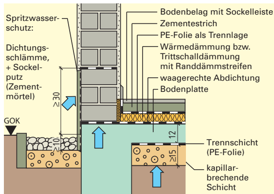
Abdichtung nicht unterkellertes Gebäude
