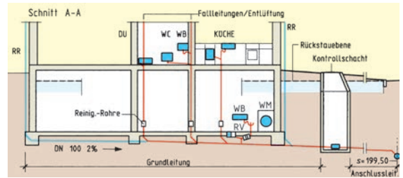
Falleitungen und Grundleitungen
