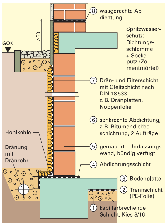
Abdichtung einer Unter-geschoss-Umfassungswand aus Mauerwerk gegen Bodenfeuchte/nicht stauendes Sickerwasser
